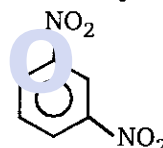
(m-dinitro benzene)
